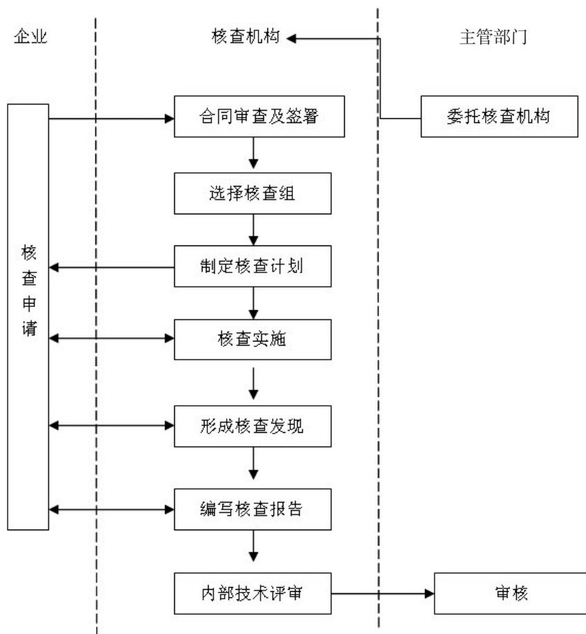
图1 核查流程
